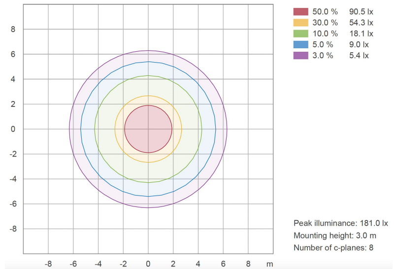
Iso-illuminance Diagram
